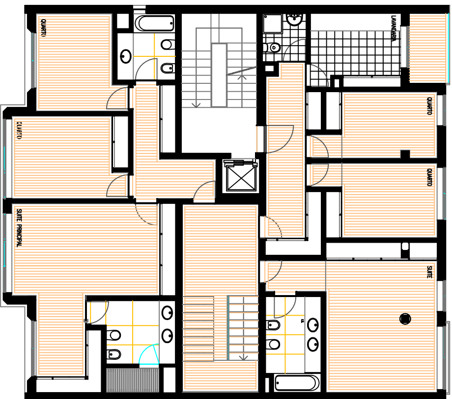
PLANTA DO 1º ANDAR
